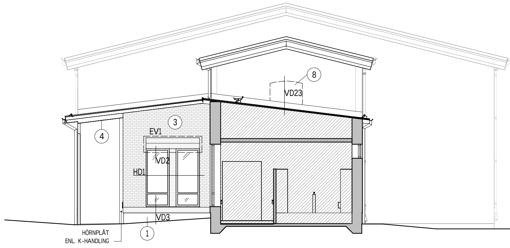
FASAD MOT NORDVÄST - ENTRÉ 1 : 100
