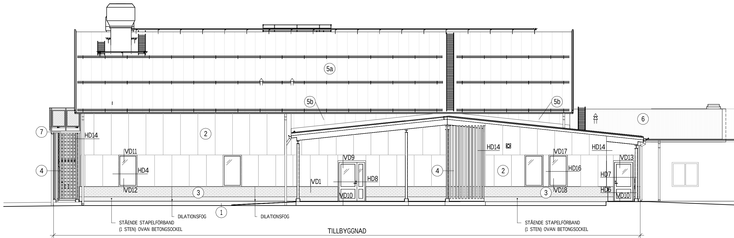
FASAD MOT NORDVÄST 1 : 100
